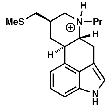
pergolide (Permax)
