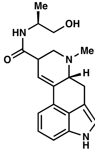
ergometrine
